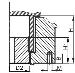
Mechanische Schnittstelle
