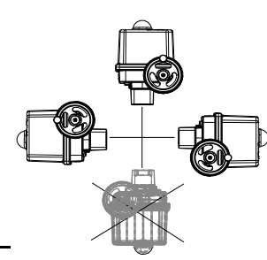
Zulässige Einbaulagen
